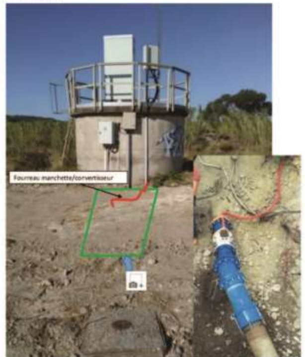
CHEVAL BLANC - LES ISLES - PUITS P5 - Débitmètre DN200 sur conduite DN250 (2 cônes fonte + assise + manchon)
